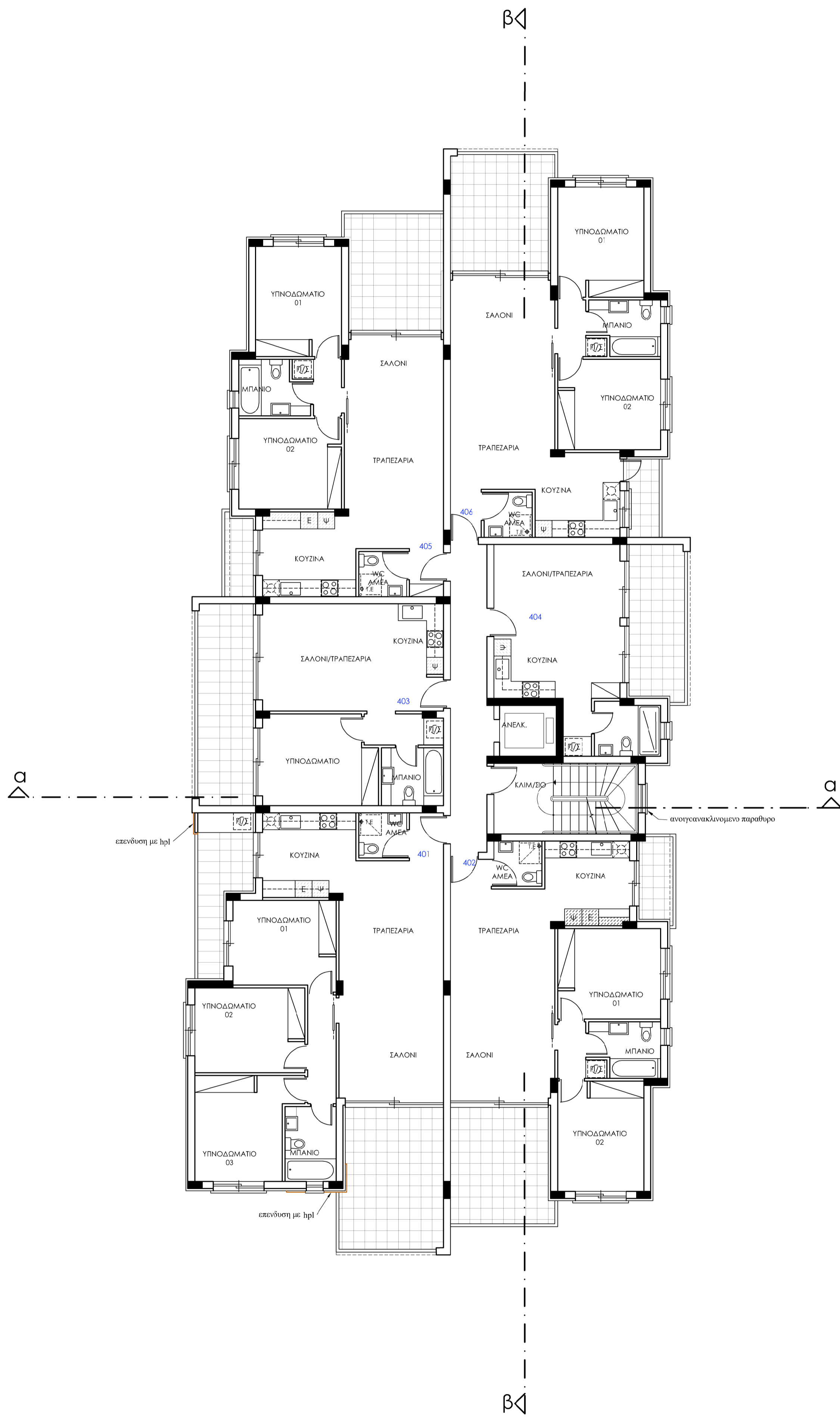
ΚΑΤΩΦΗ 4ου ΟΡΟΦΟΥ ΠΟΛΥΚΑΤΟΙΚΙΑ BLOCK B
