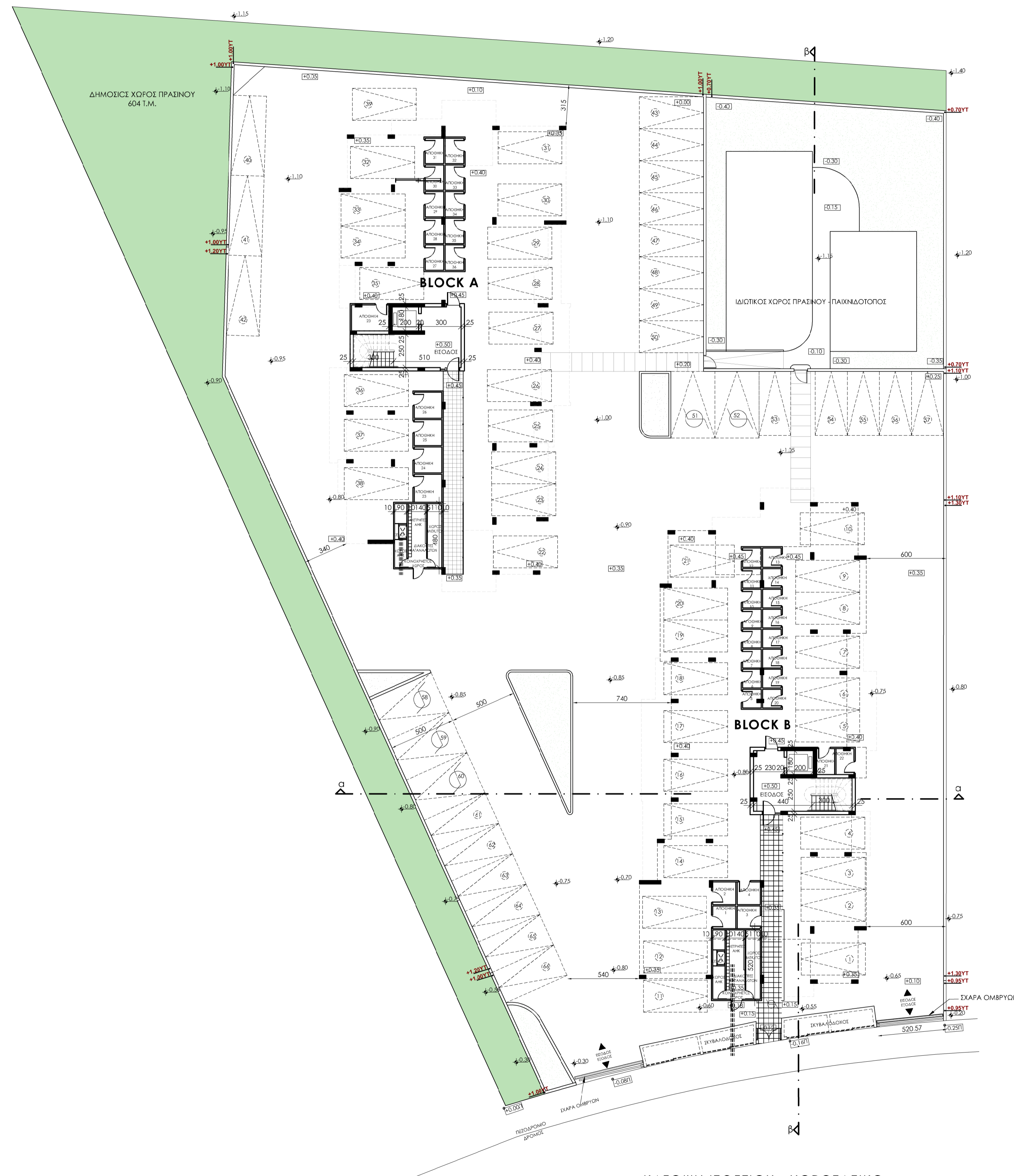
ΚΑΤΟΨΗ ΙΣΟΓΕΙΟΥ - ΧΩΡΟΤΑΞΙΚΟ
