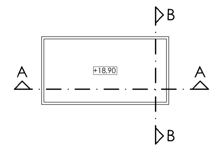
ΚΑΤΩΦΗ ΟΡΟΦΗΣ ΚΛΙΜΑΚΟΣΤΑΣΙΟΥ ΠΟΛΥΚΑΤΟΙΚΙΑ BLOCK A
